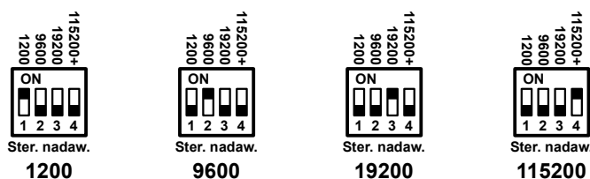
Rysunek 6: Ustawienia sterowania nadawaniem interfejsu RS-485/RS-422/2xRS-485
