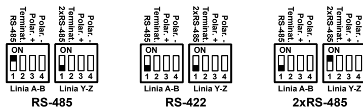
Rysunek 3: Ustawienia trybu pracy interfejsu RS-485/RS-422/2xRS-485
