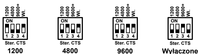
Rysunek 7: Ustawienia sterowania linią CTS interfejsu RS-232
