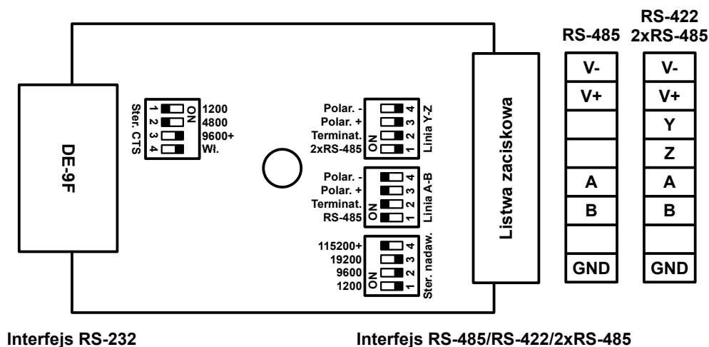
Rysunek 2: Rozmieszczenie przełączników i złączy
