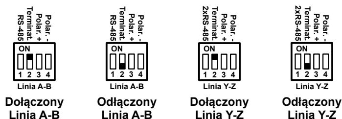
Rysunek 4: Ustawienia terminatorów linii interfejsu RS-485/RS-422/2xRS-485
